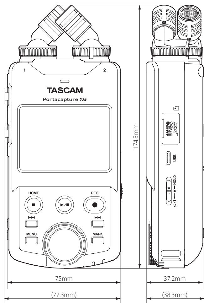
18-2 外形尺寸图
